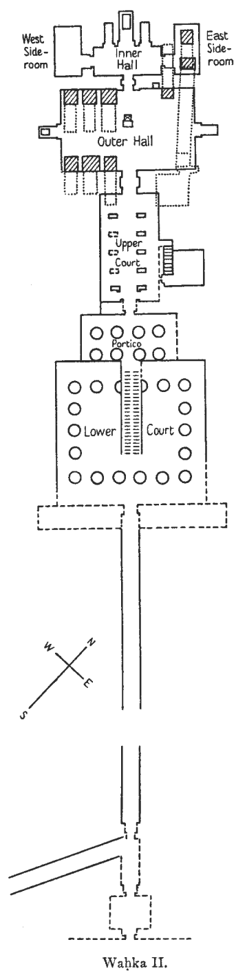
QAW EL-KEBÎR. After STECKEWEH, Die Fürstengräber von Qaw , Plans I-VI.
